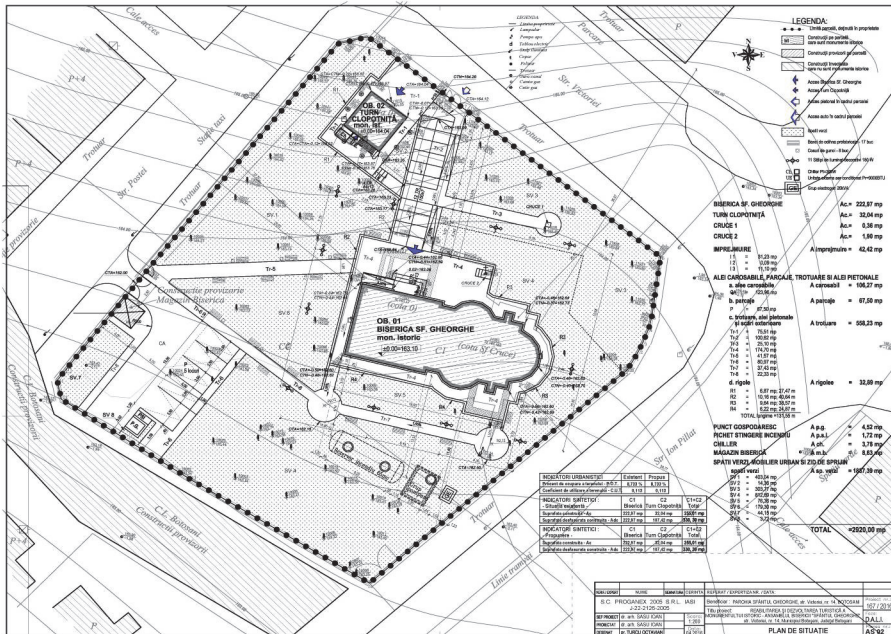
Fig. 1. Planul de încadrare în zonă și planul bisericii Sf. Gheorghe din Botoșani
