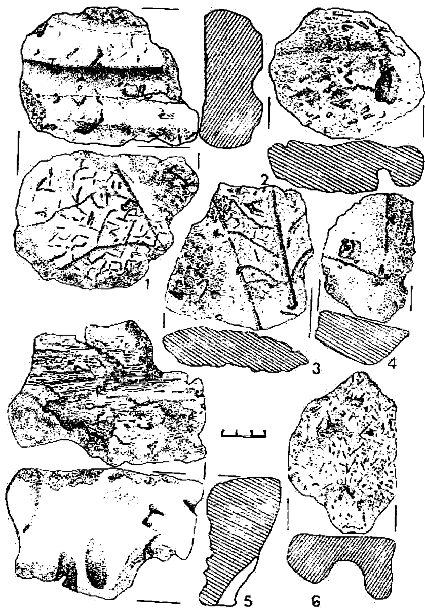
Fig. 3. Chetrești-Capul Dealului. Faza A. Fragmente de materiale de construcție din lut cu resturi vegetale. L 2 1-2,4-5; în strat 3; L 1 6.
